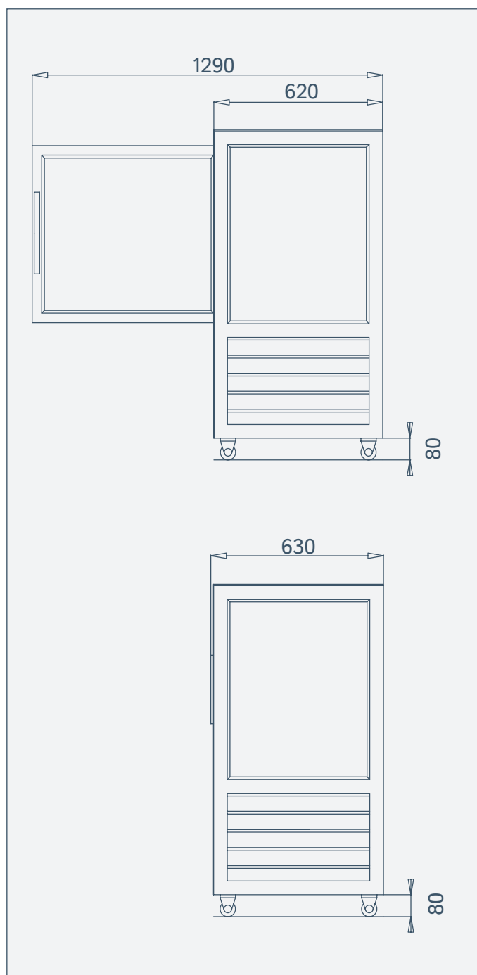
VISTA LATERALE
